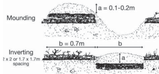
Figure 10 En haut, le scarifiage par monticules ( mounding ) et en bas, le scarifiage par inversion ( inverting ) (tiré de Hallsby et Örlander, 2004)
